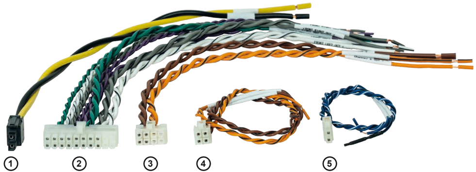
Abb. 2: Übersicht Anschlusskabel
