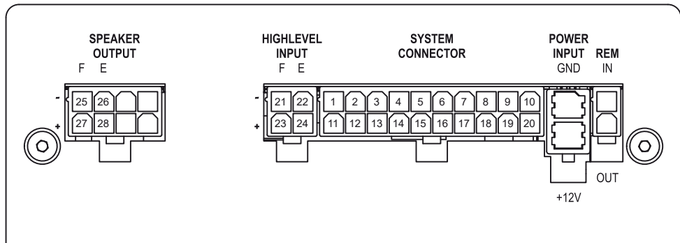
Abb. 1: Pinbelegung UP 6DSP
